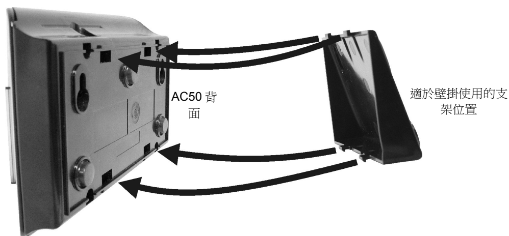
圖 4. 壁掛使用時的 AC50 背面支架安裝
